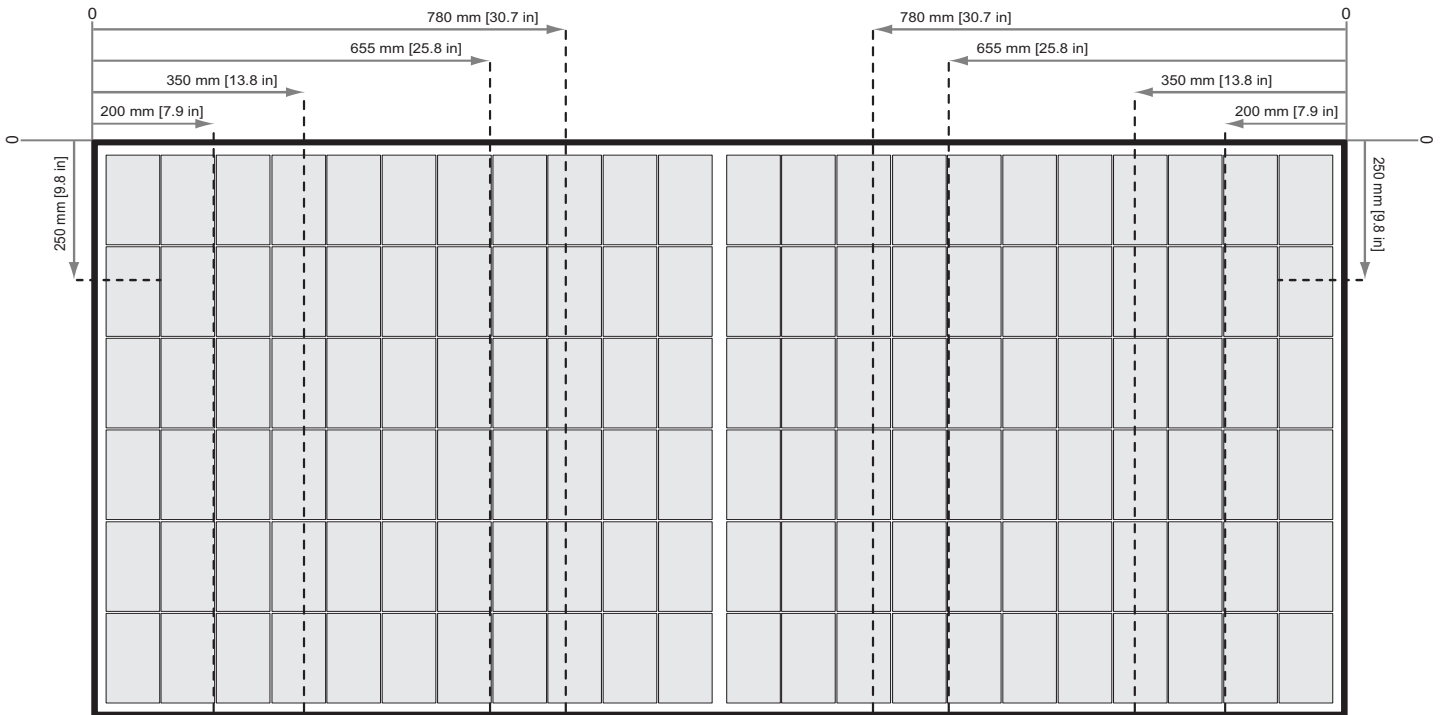
Abb. 6: Befestigen von REC Alpha 72 Serie Modulen auf durchlaufenden Schienen parallel zur kurzen Seite des Moduls
