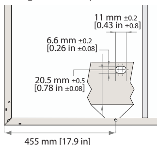
Abb. 8: Montagelöcher: REC Alpha Serie
