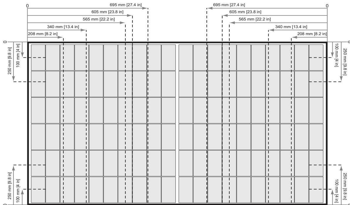
Abb. 5: Befestigen von REC Alpha Serie Modulen mit Kurzschienen
