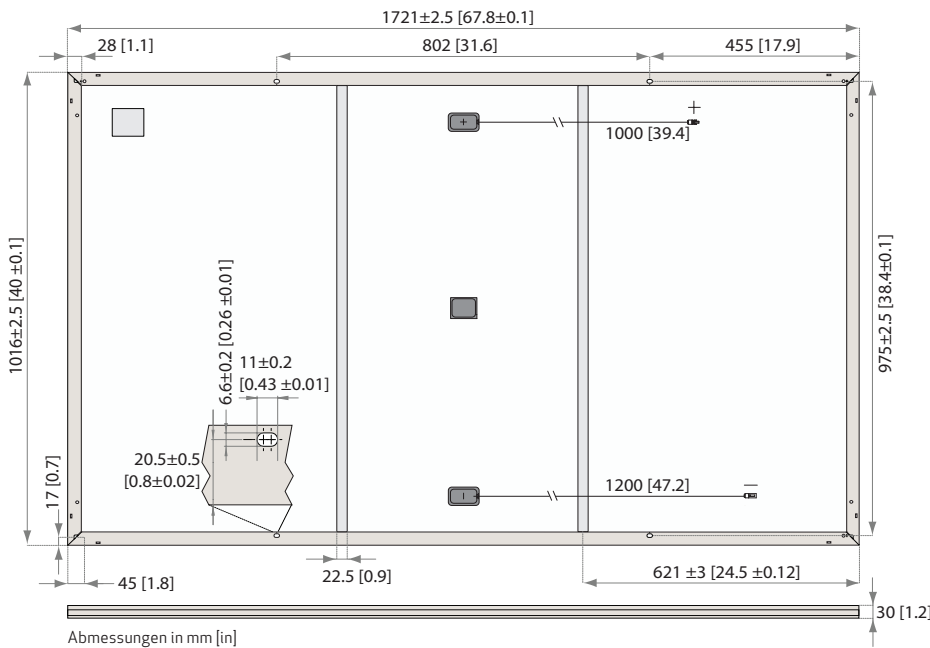
Abb. 16: Abmessungen: REC Alpha Serie
