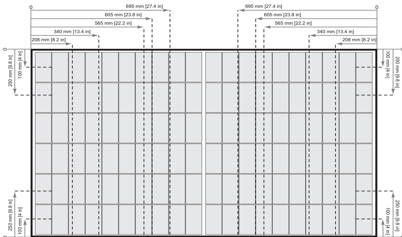
Abb. 3: Befestigen von REC Alpha Serie Modulen auf Schienen parallel zur kurzen Seite des Moduls
