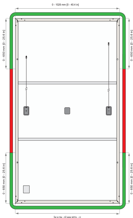
Abb. 20: MLPE-Geräte Installationsbereiche: REC Alpha 72 Serie
