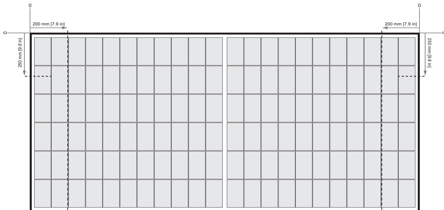
Abb. 7: Befestigen von REC Alpha 72 Serie Modulen auf Kurzschienen parallel zur kurzen Seite des Moduls
