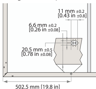
Abb. 9: Montagelöcher: REC Alpha 72 Serie
