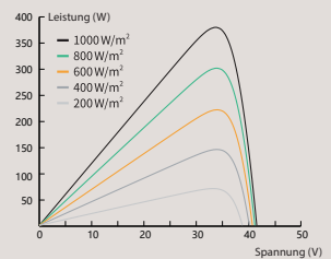
Leistung-Spannungs-Kennlinie (380 W)
