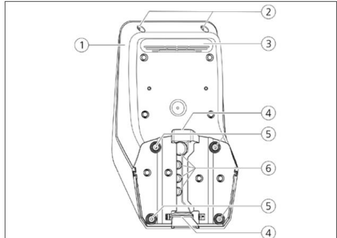
Rückansicht
