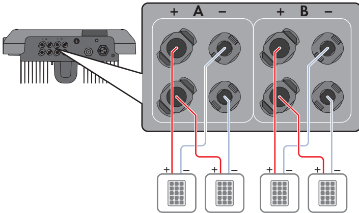
Abbildung 9: Übersicht des Anschlusses bei Normalbetrieb
