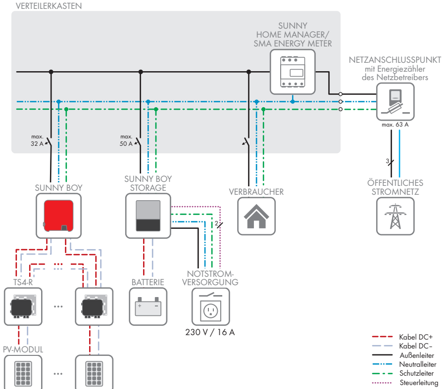
Abbildung 3: Verschaltungsübersicht (Beispiel)
